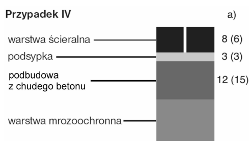
2.4. Konstrukcja nawierzchni dla kategorii ruchu R_3 – grubość warstwy w [cm]
