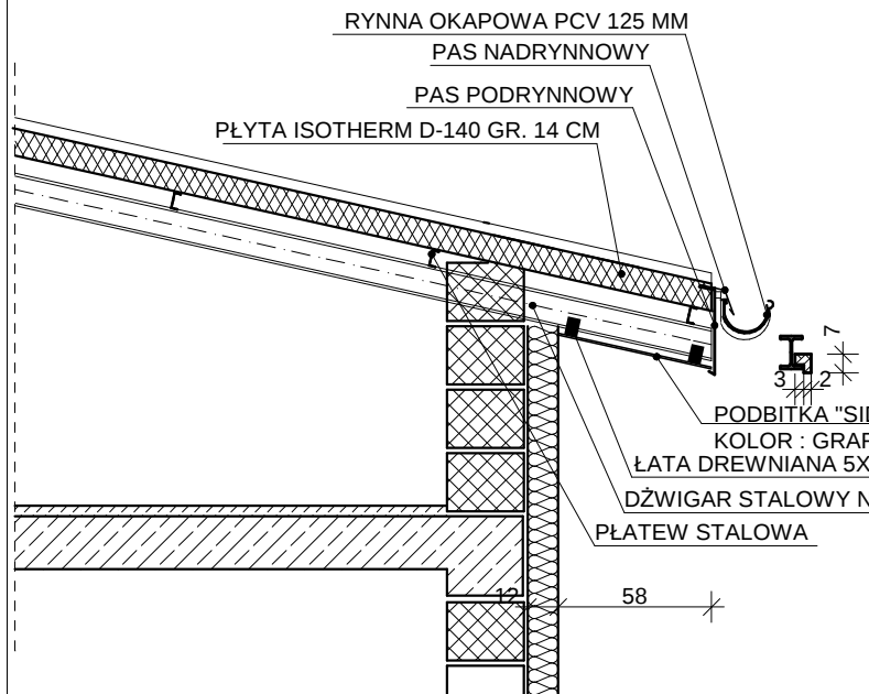
SZCZEGÓŁ "A" SKALA 1:20
