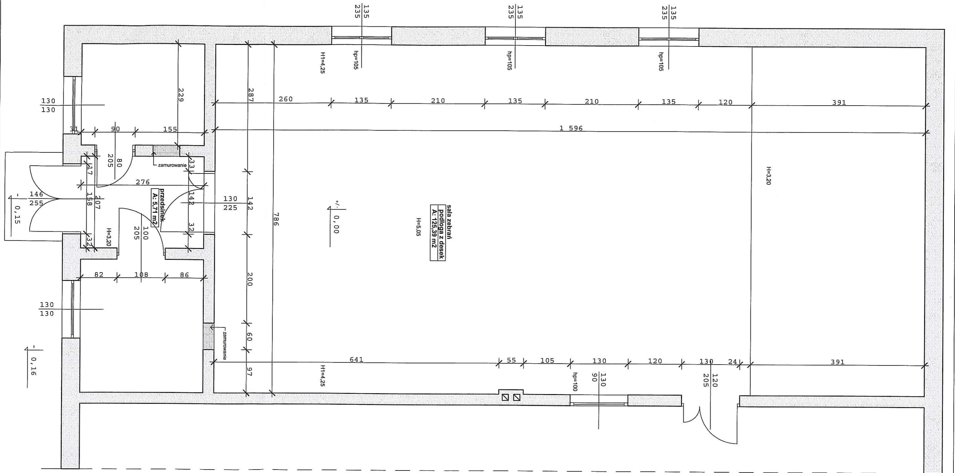
RZUT PRZYZIEMIA 1:50 (fragment) projekt
